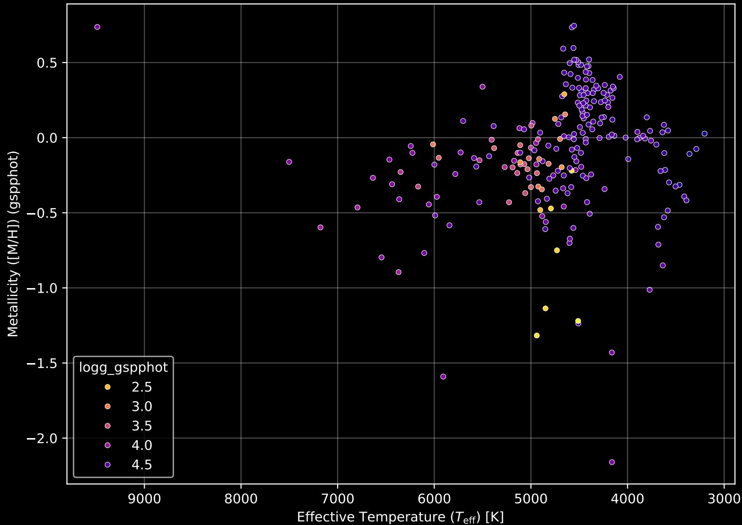
APOGEE DR17 Field: [264-33-C] Stellar Population Parameters (n= 224)
